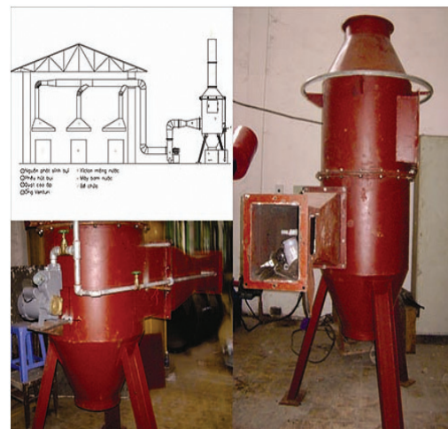
Thiết bị lọc bụi, khí cho các làng nghề
